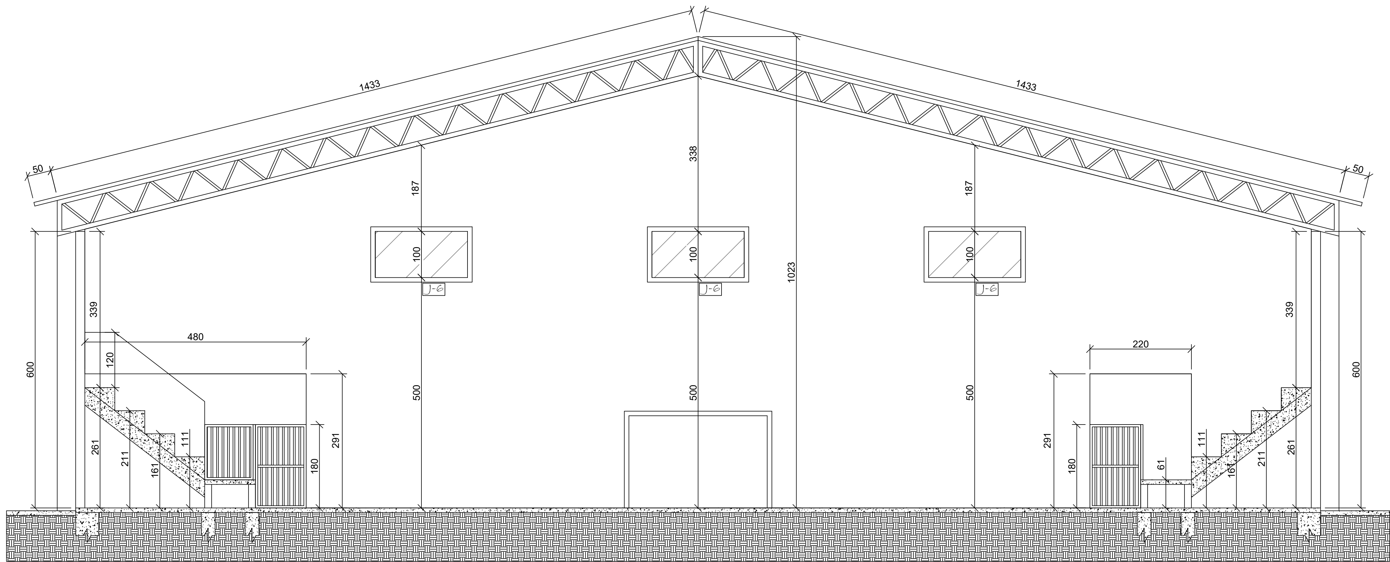
CORTE BB
