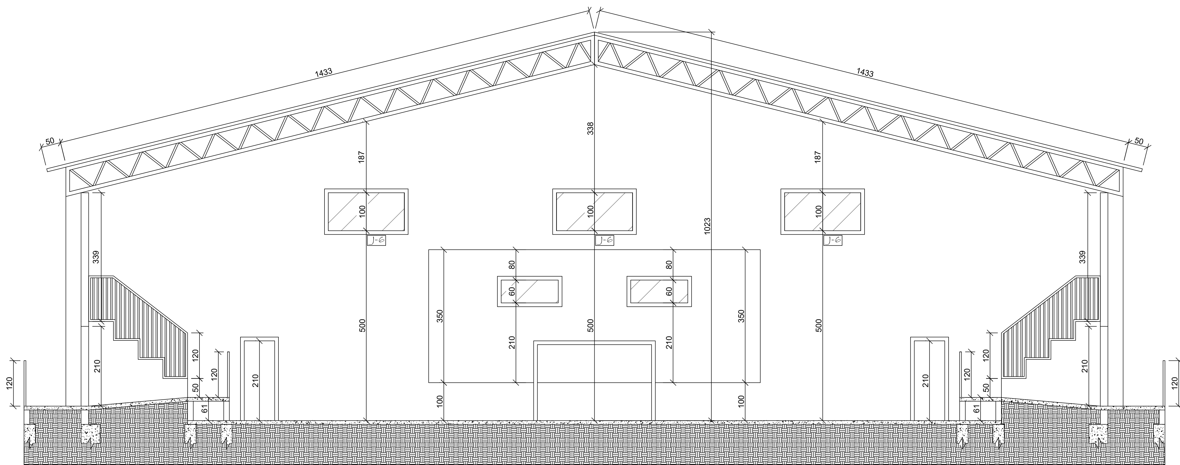
CORTE CC
