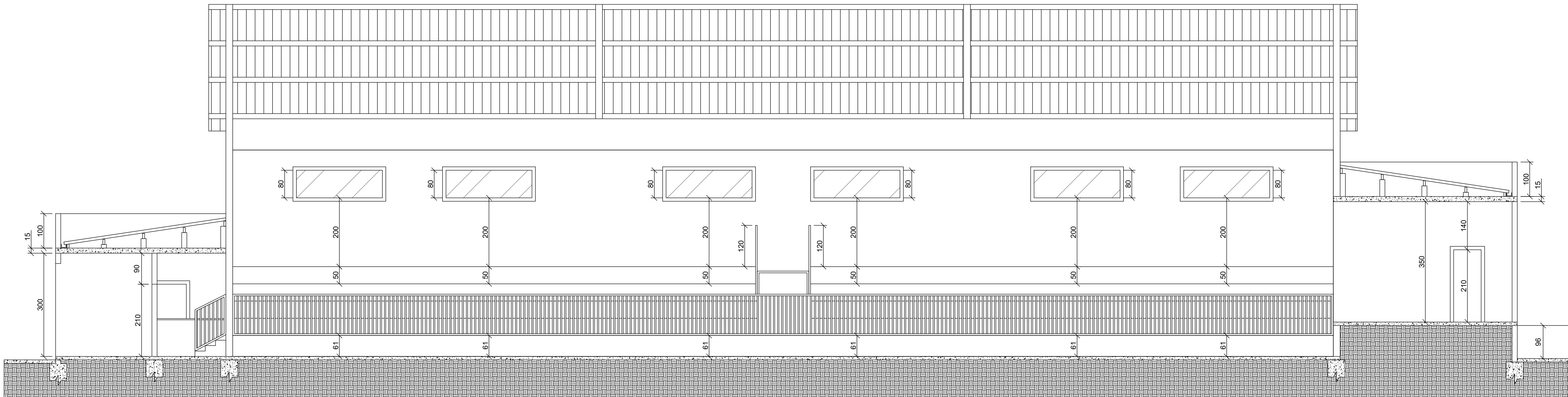
CORTE AA
